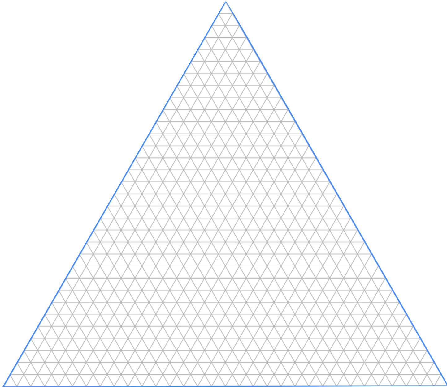
Sierpinski Triangle Grid
